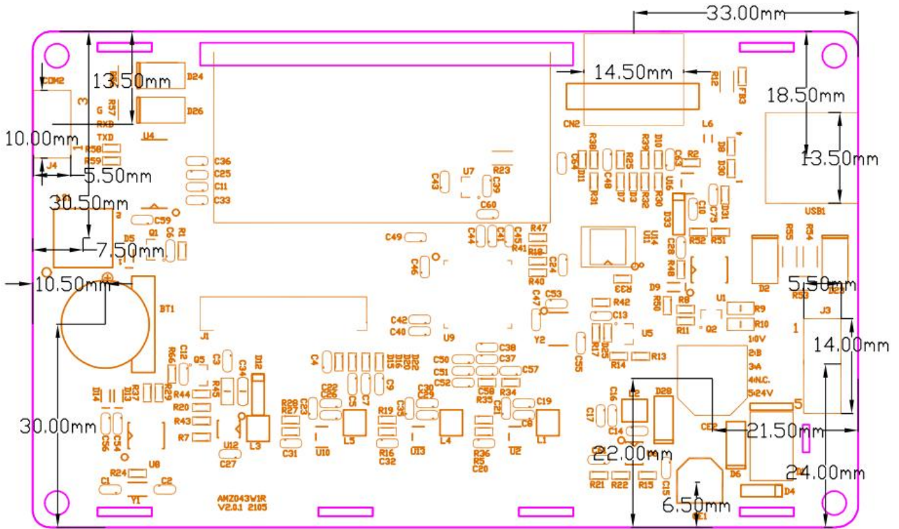
AMZ043 背面图
